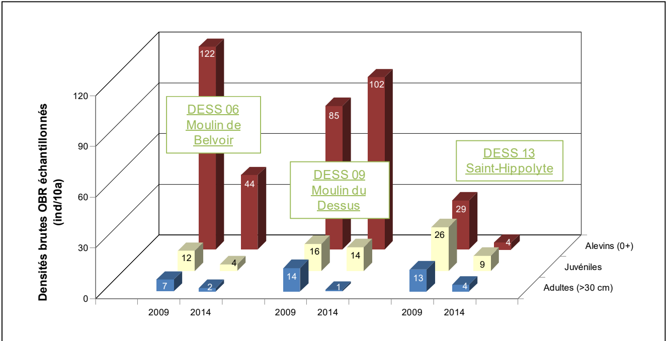
Figure 2.14. : Densités surfaciques des différents stades de développement de l'ombre commun sur le Dessoubre
