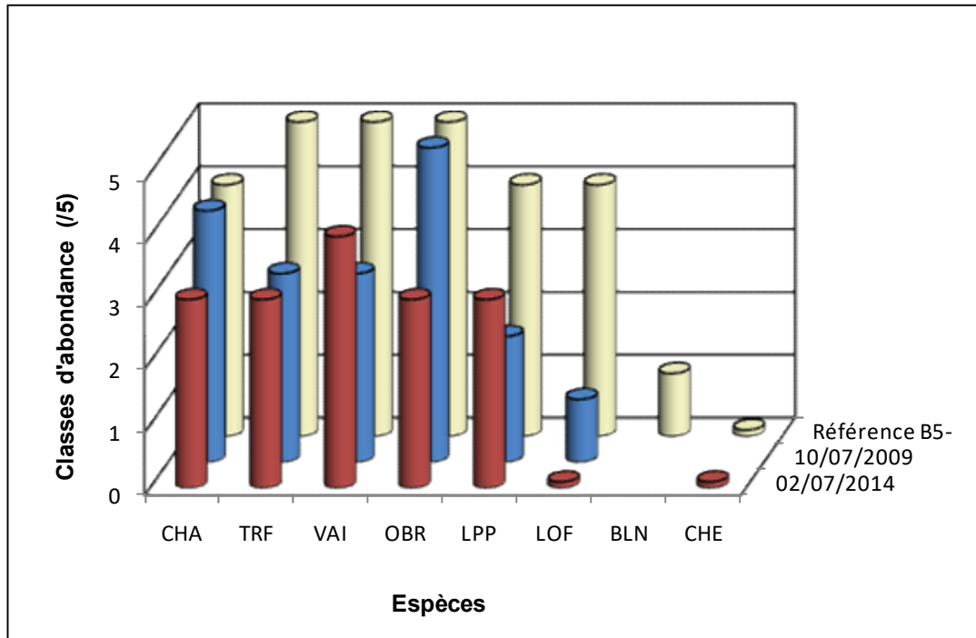
Figure 2.8. : Confrontation entre les peuplements observés et théoriques sur la station DESS 09
