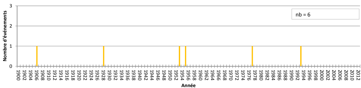
Chronologie des événements d'intensité III à Premeaux-Prissey (1900-2012)
