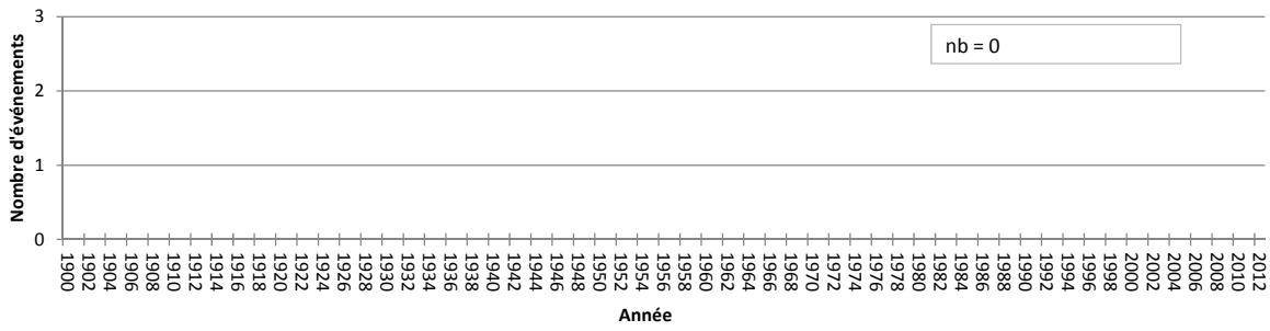
Chronologie des événements d'intensité V à Meursault (1900-2012)
