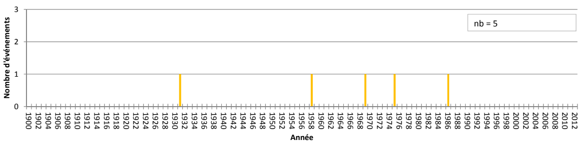
Chronologie des événements d'intensité III à Monthelie (1900-2012)
