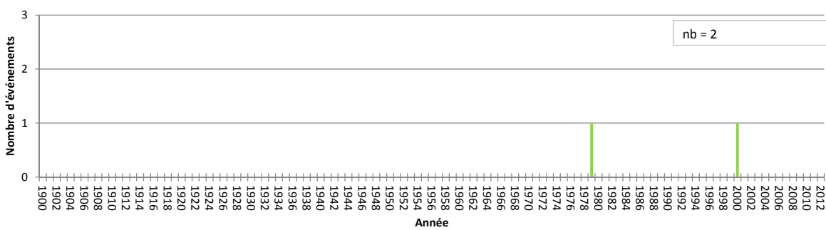
Chronologie des événements d'intensité II à Monthelie (1900-2012)
