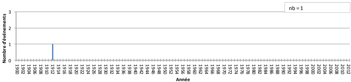
Chronologie des événements d'intensité I à Chassagne-Montrachet (1900-2012)
