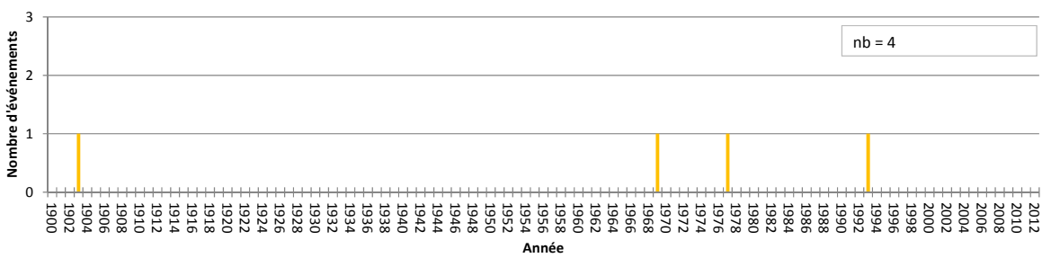
Chronologie des événements d'intensité III à Vosne-Romanée (1900-2012)
