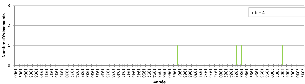
Chronologie des événements d'intensité II à Savigny-lès-Beaune (1900-2012)
