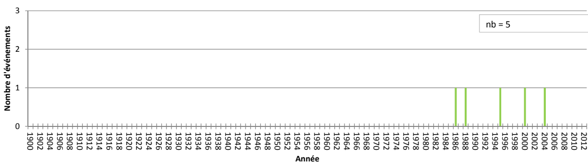
Chronologie des événements d'intensité II à Meursault (1900-2012)
