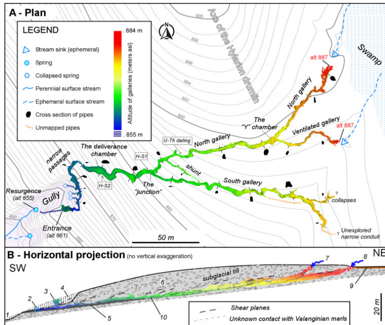
Figure : Plan et coupe de la grotte d'Hylarion (Durllet et al., 2024)
