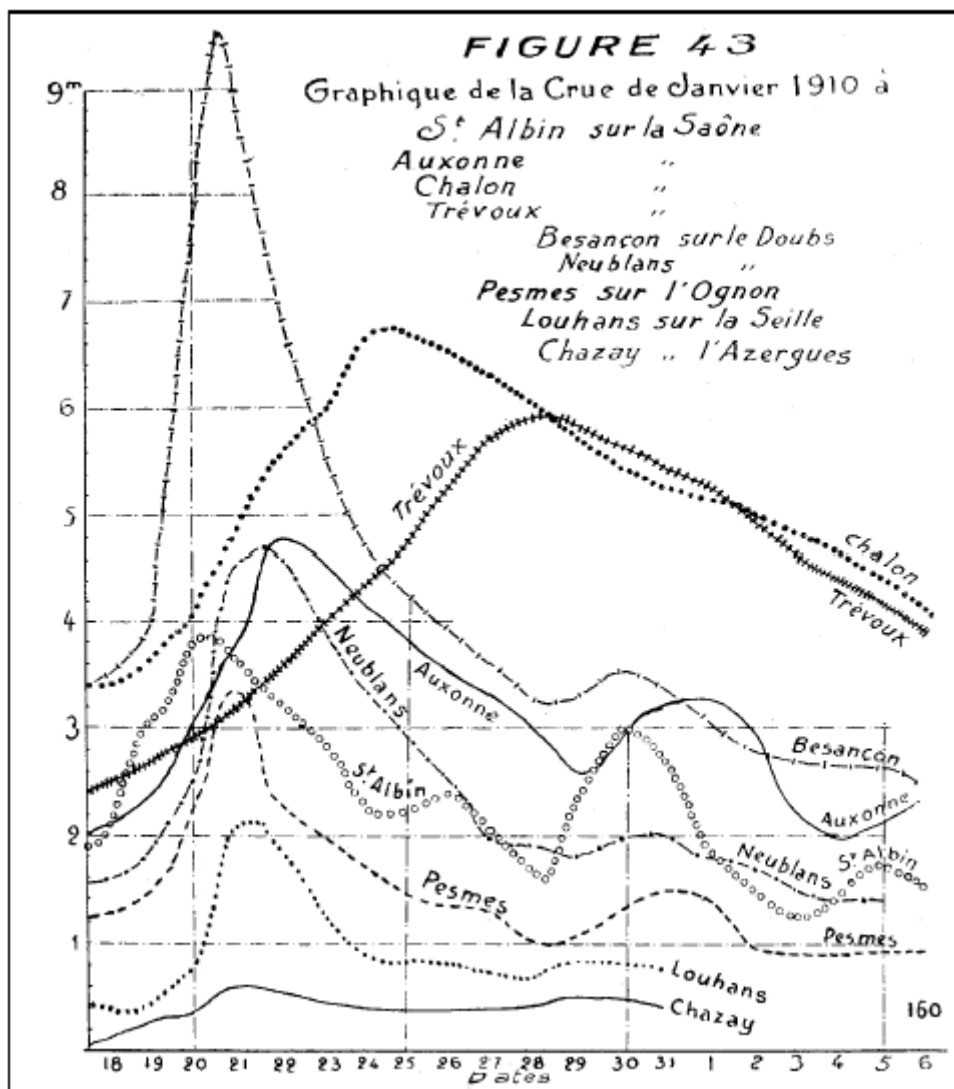
Hydrogrammes des différents rivières affluants du Rhône amont
